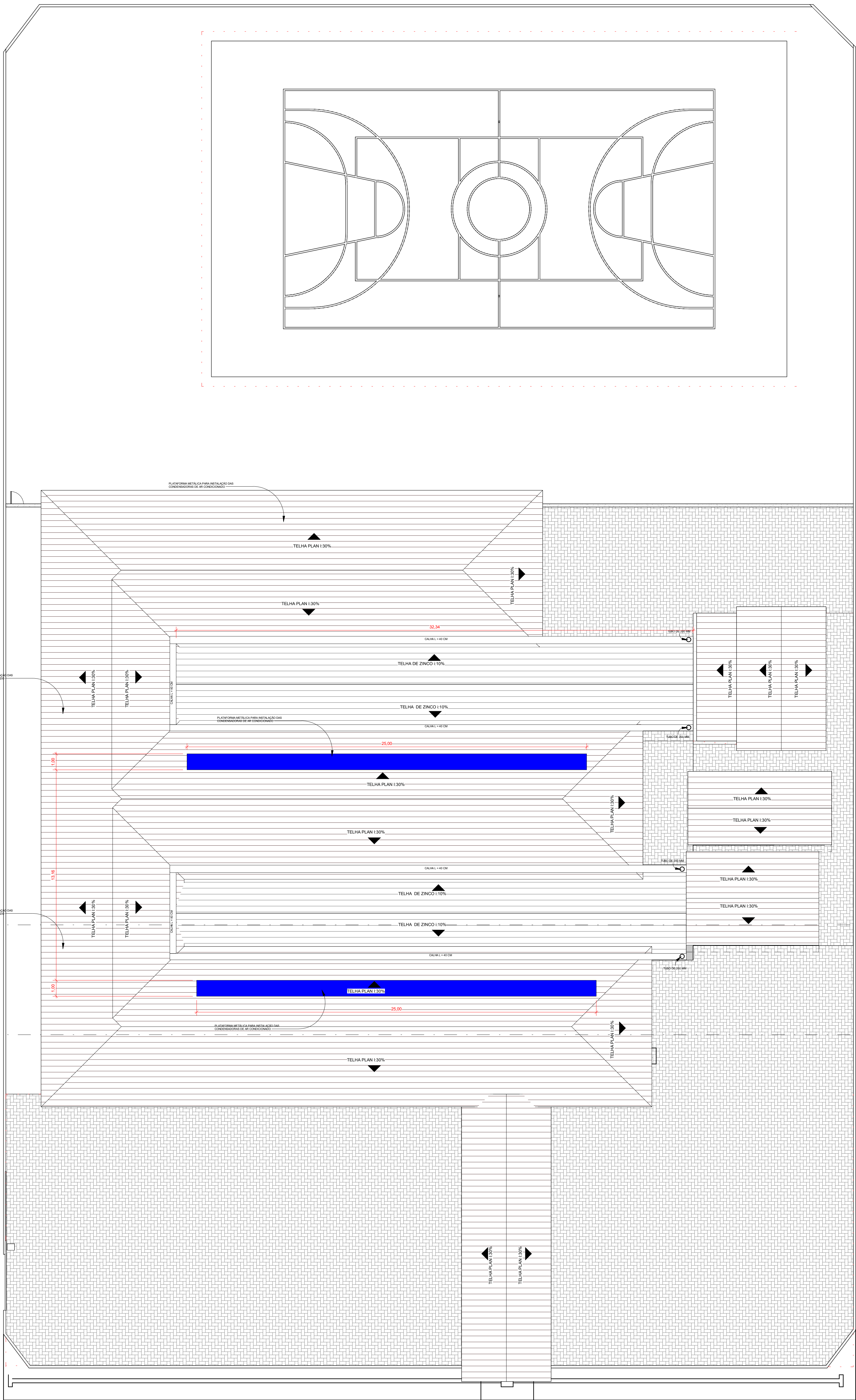
PLANTA DE COBERTURA ESCALA: 1 : 125
